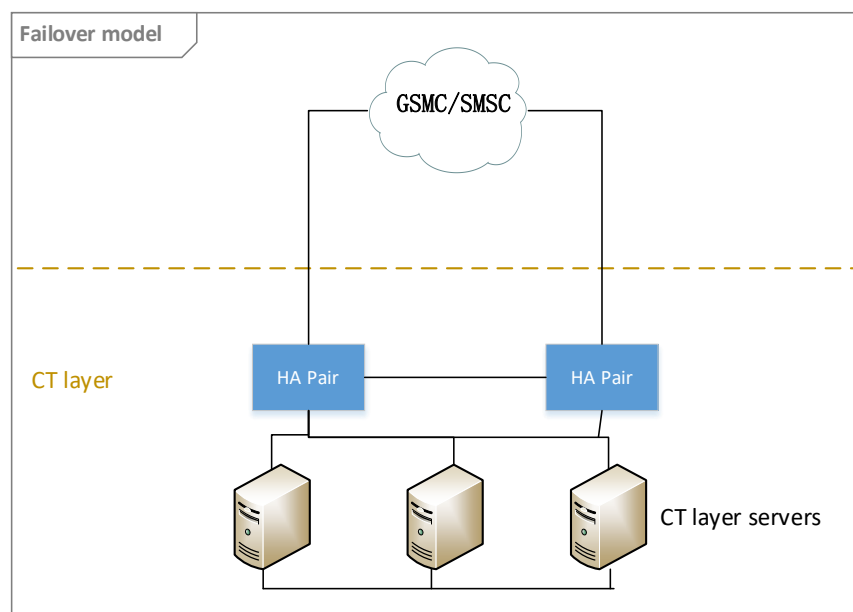
Hình 3: Mô hình dự phòng tầng CT
